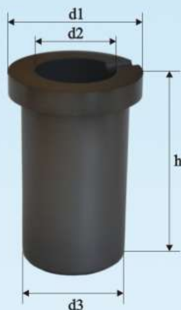
Тигель графитовый G.GM.1000A 1 кг стакан малый
